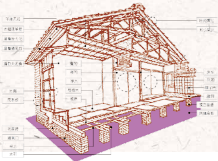
321 巷建築構造剖面圖
